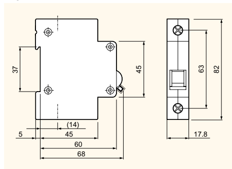
Figura 1 : Tipo BKN & BKN-c
