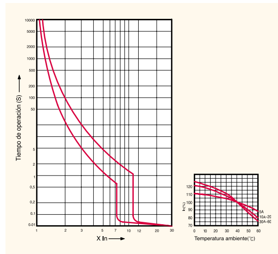
Curva 2 : Tipo BFN
